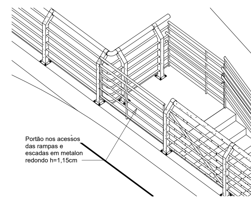
6 Det dos guarda corpo
