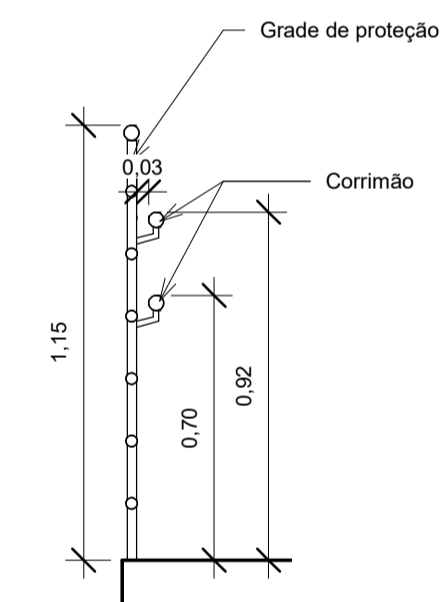
9 Det. Guarda corpo mod. 02 1 : 20 Guarda corpo das escadas e rampa
