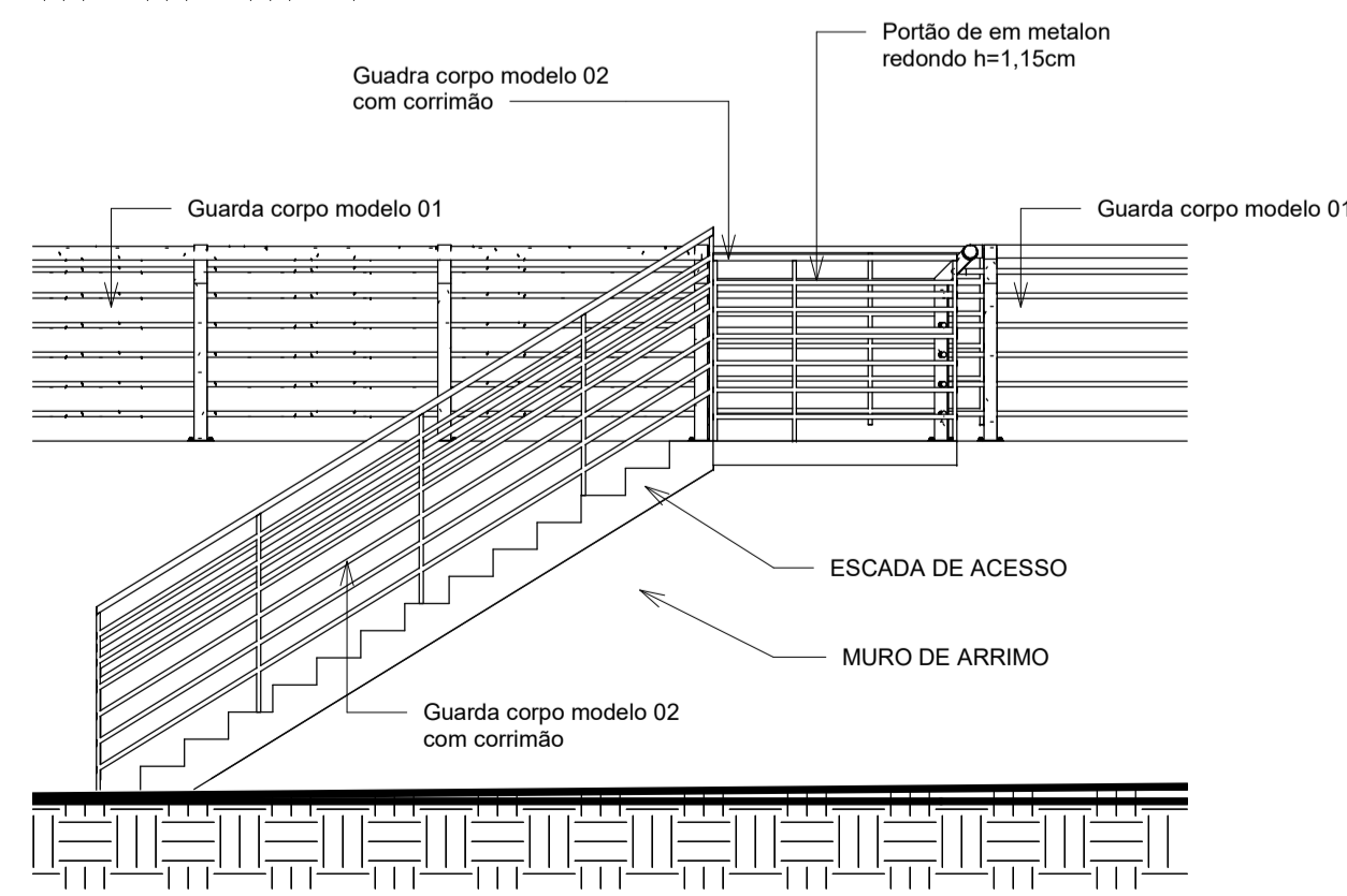
7 VISTA DA ESCADA 1 : 50
