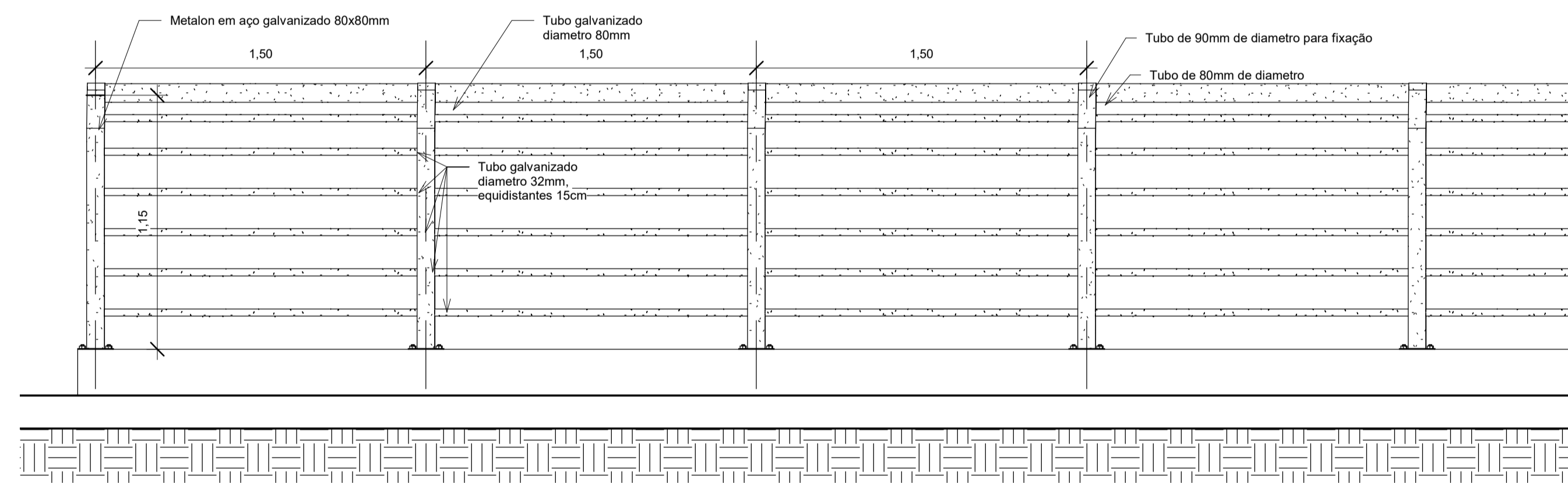
2 Det. Guarda corpo mod. 01 1 : 20
