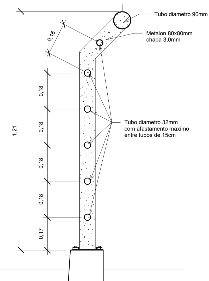
1 Corte grade mod. 01 1 : 10
