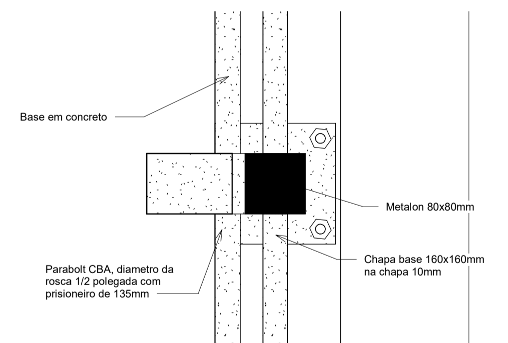
4 Detalhe da base de fixação 1 : 5
